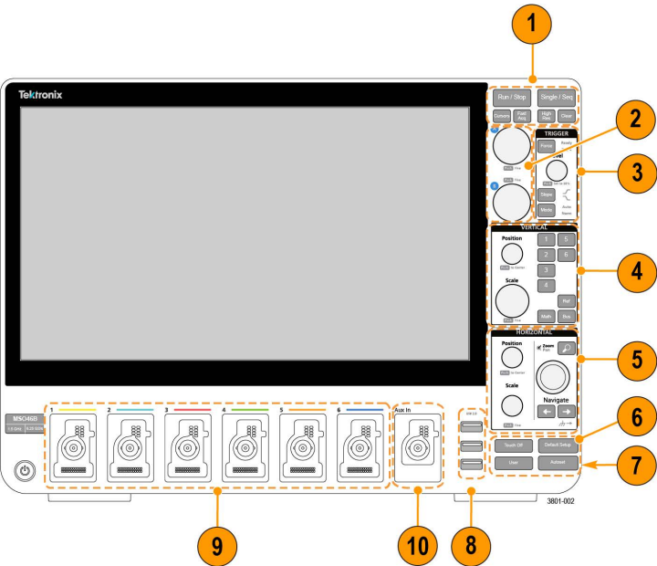
图3: 4 系列 BMSO 控件
