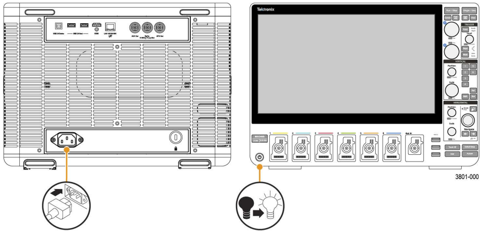
图1: MSO44B 和 MSO46B 电源线连接器和电源待机开关
