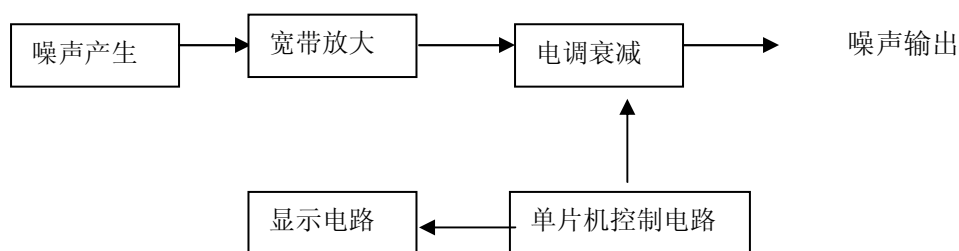
图 3 噪声源功能框图
