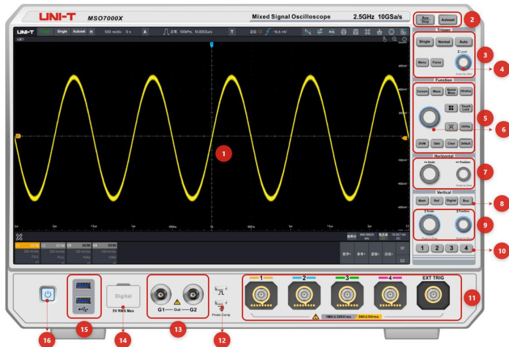
示波器前面板
