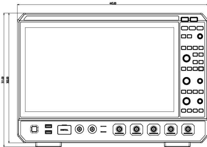
主视图
