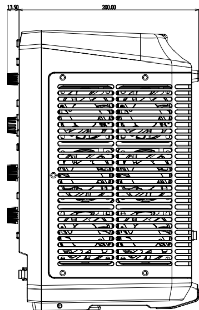
侧视图
