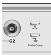
探头补偿信号连接片和接地端
