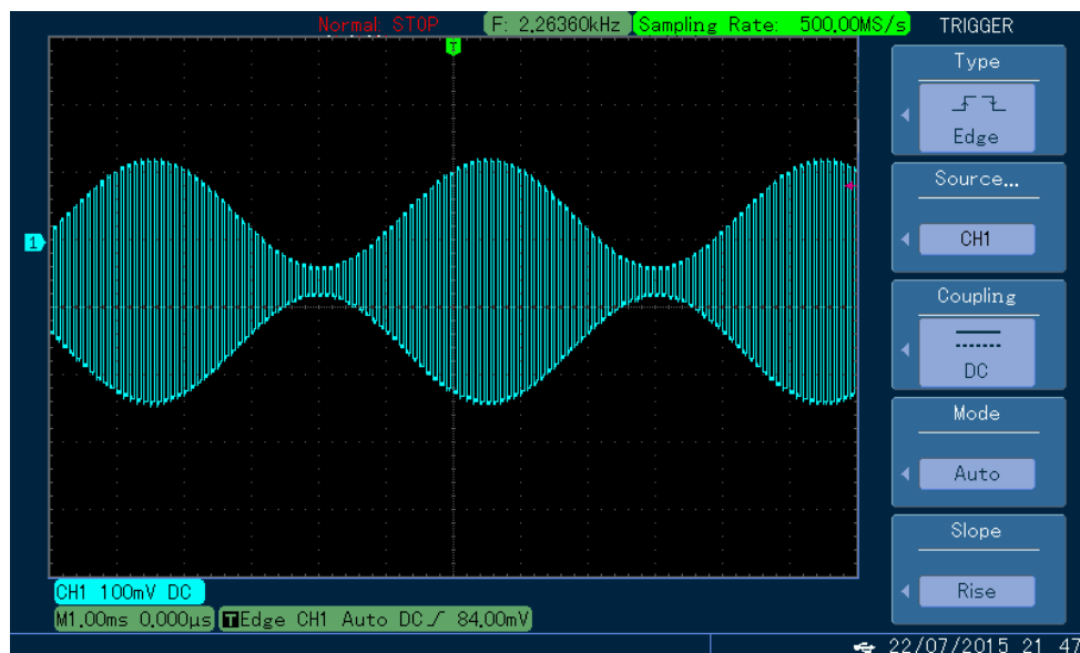
图 4-13 示波器观察调幅波形
