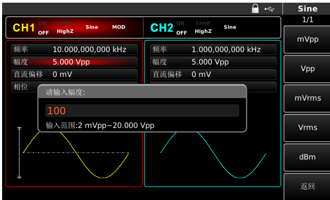
图 4-21 设置载波幅度
