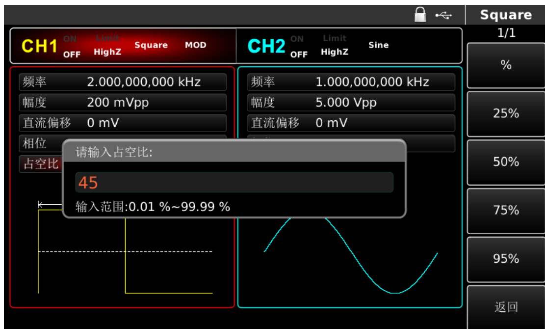
图 4-105 设置载波占空比
