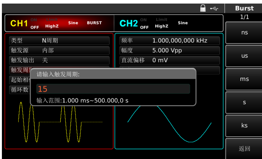
图 4-147 设置脉冲周期
