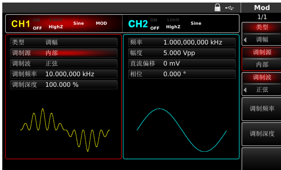
图 4-3 选择调制源
