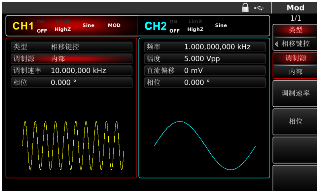
图 4-58 选择调制源
