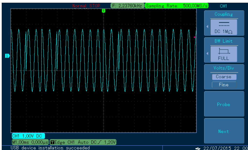
图 4-72 示波器观察双相移键控波形
