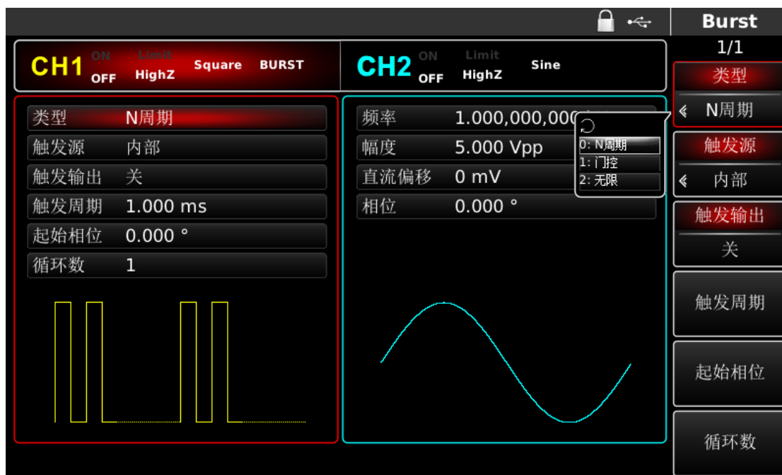
图 4- 143 设置为 N 循环功能
