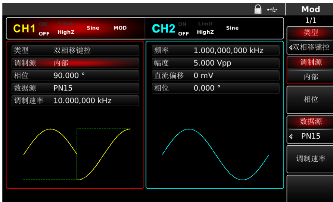
图 4-66 选择调制源
