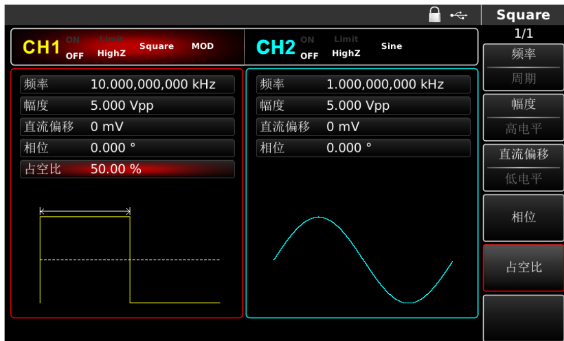
图 4-8 选中载波占空比
