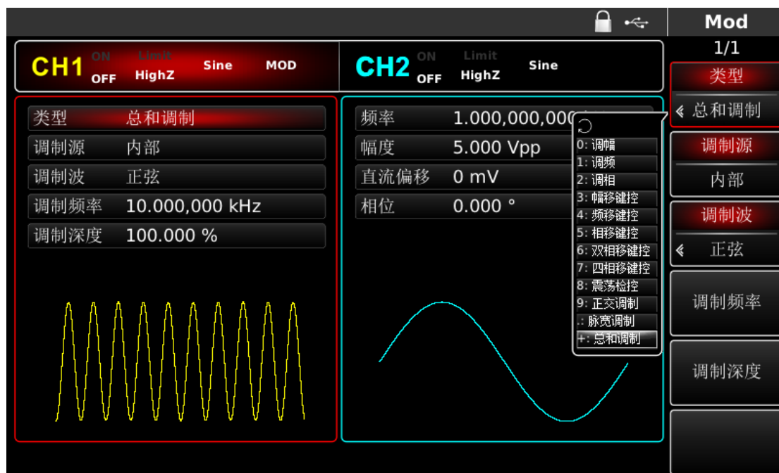
图 4-102 选中总和调制功能
