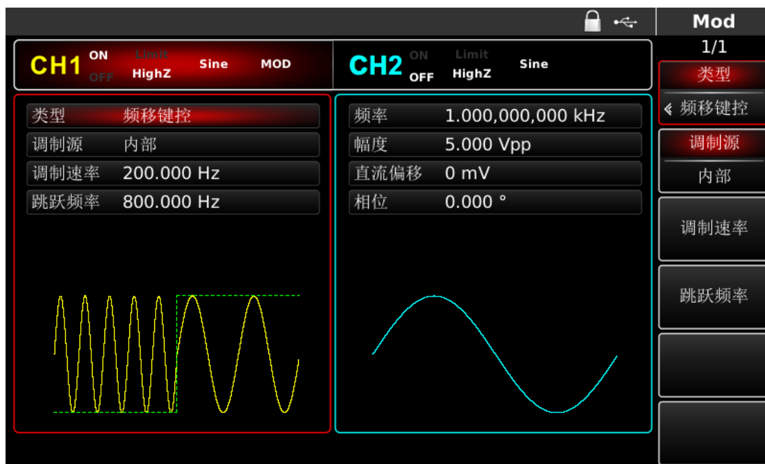
图 4-54 启用通道输出
