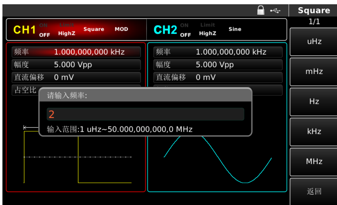
图 4- 104 设置载波参数
