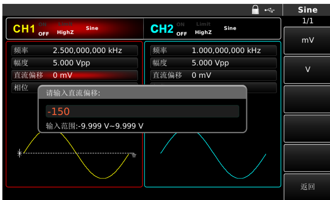
图 3-4 设置偏移电压
