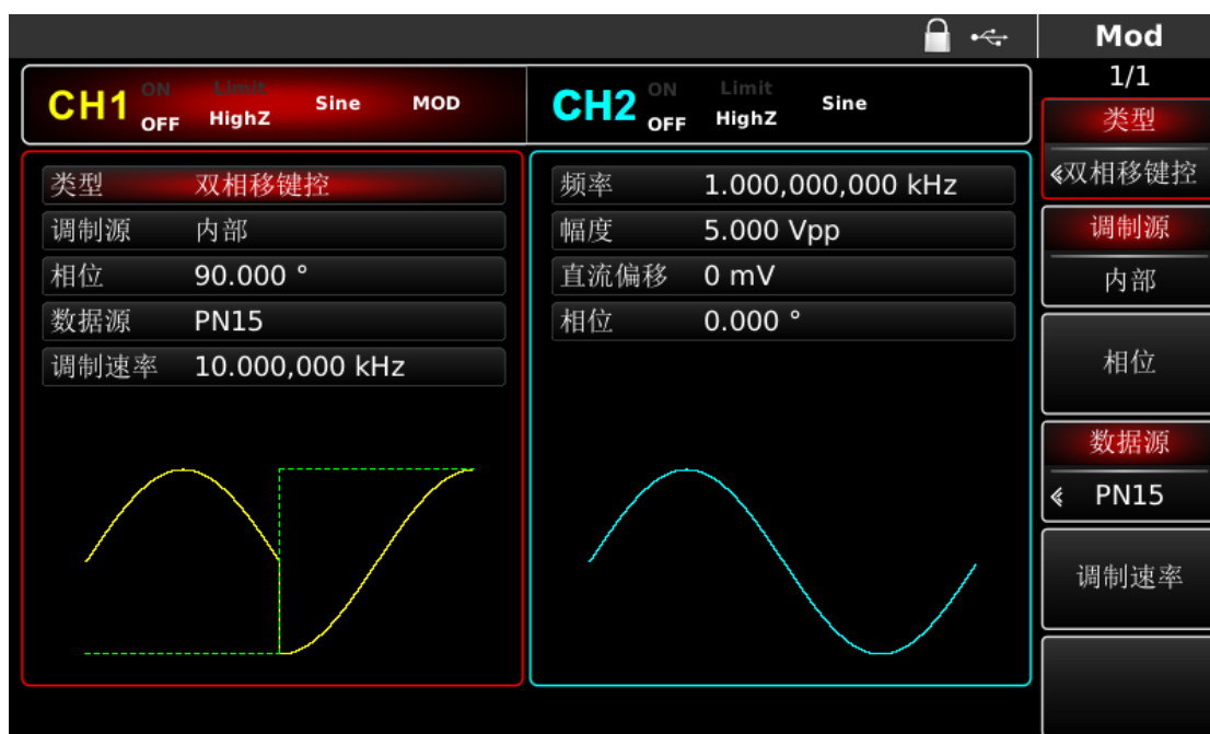
图 4-69 设置调制参数
