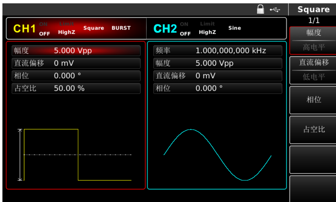
图 4-136 选择波形
