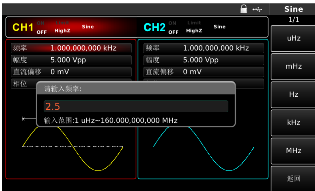
图 3-2 设置频率
