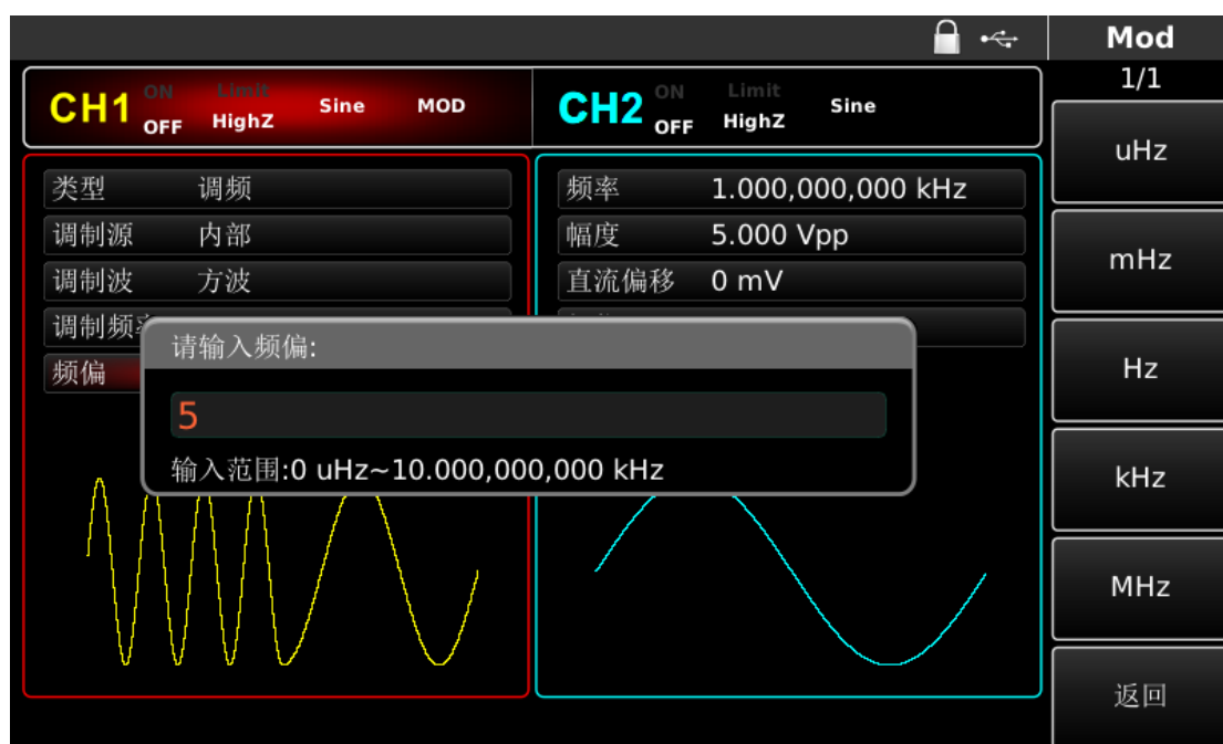
图 4-23 设置频率偏差
