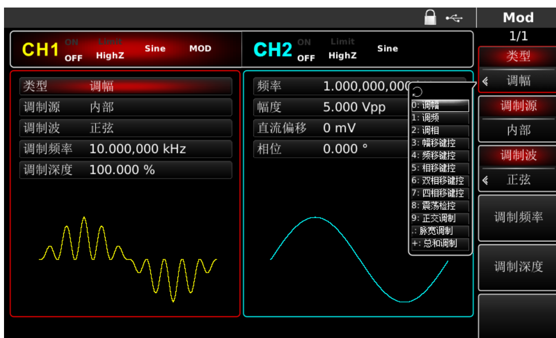
图 4-1 选中调幅功能
