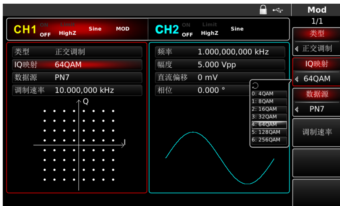
图 4-96 设置调制参数
