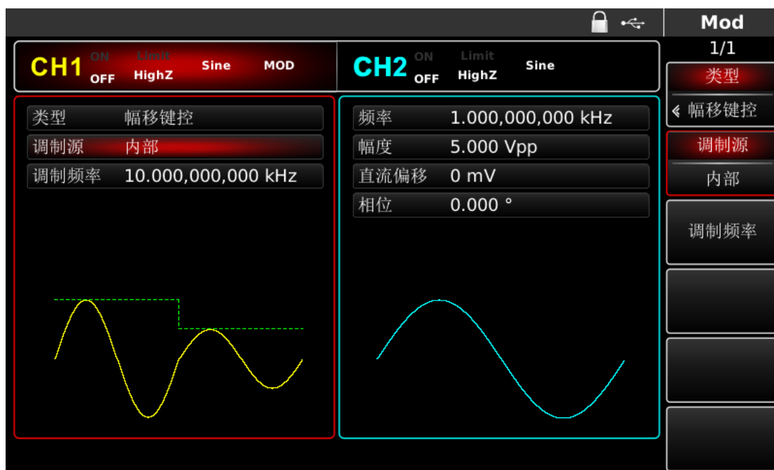
图 4-39 选中调制源
