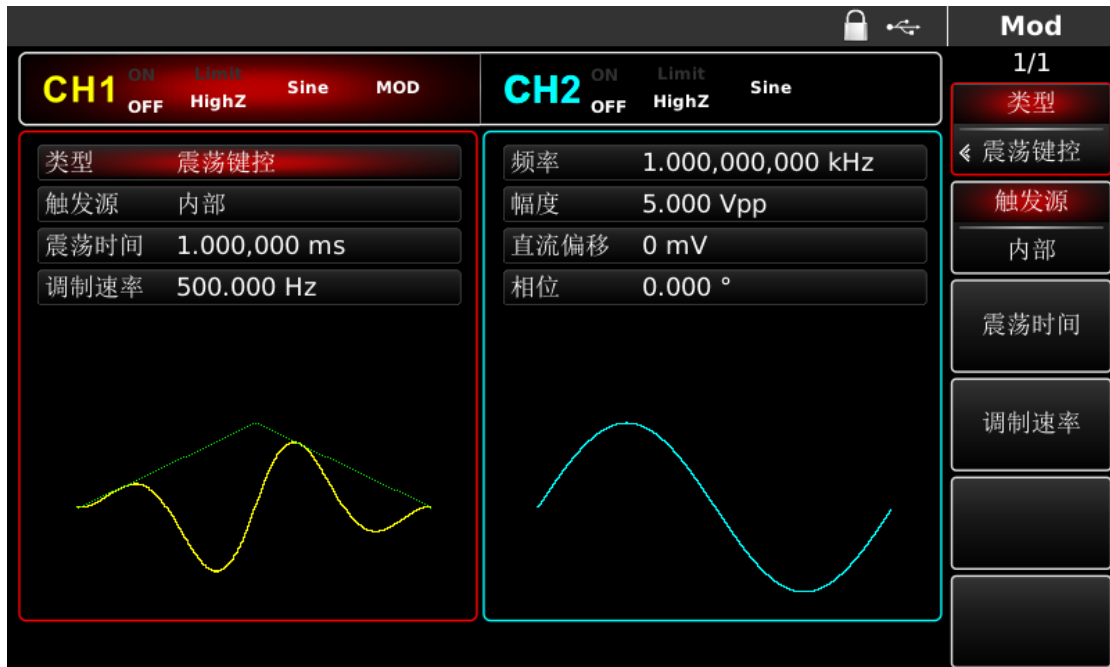
图 4-85 选择调制源
