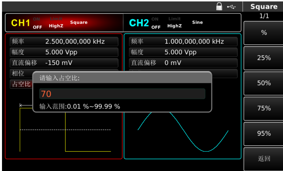
图 3-5 设置占空比
