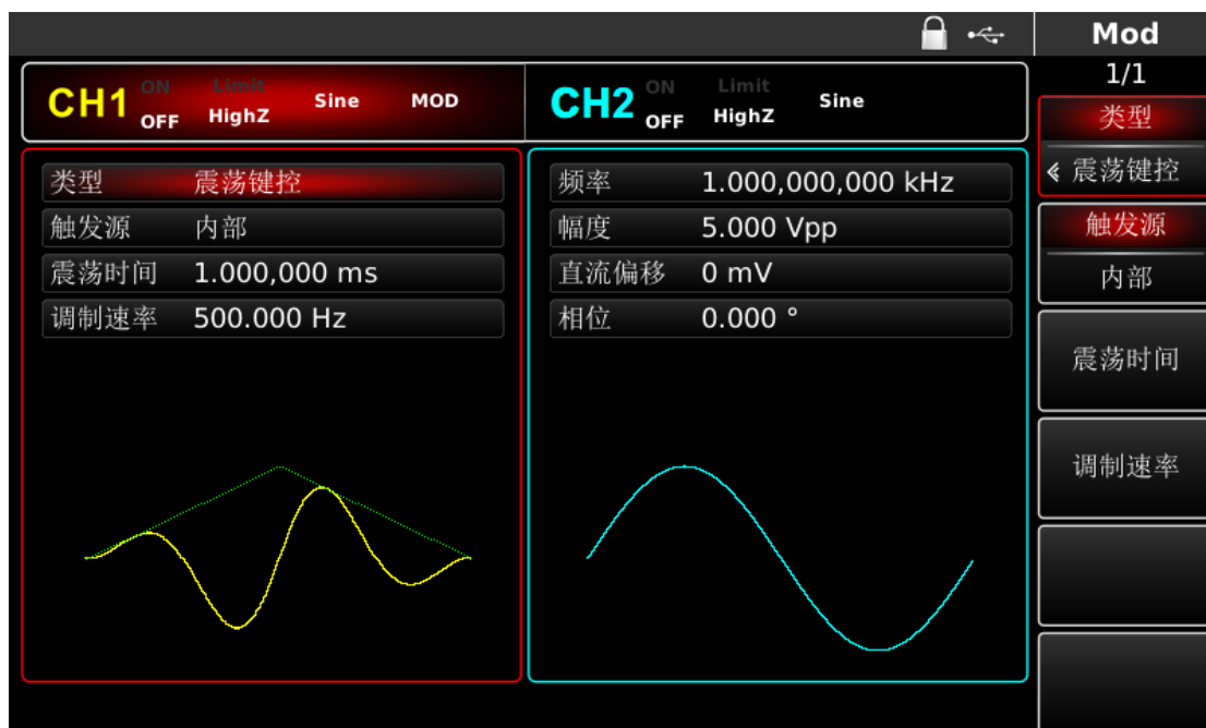
图 4-84 选择调制源
