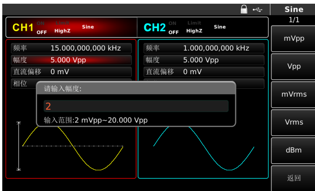
图 4-42 设置载波幅度
